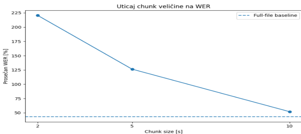
Слика 5. Утицај chunk величине на WER
