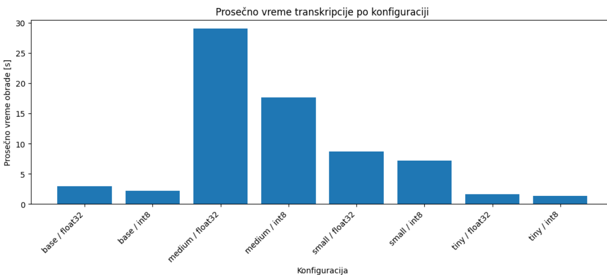
Слика 4. Просечно време транскрипције по конфигурацији
