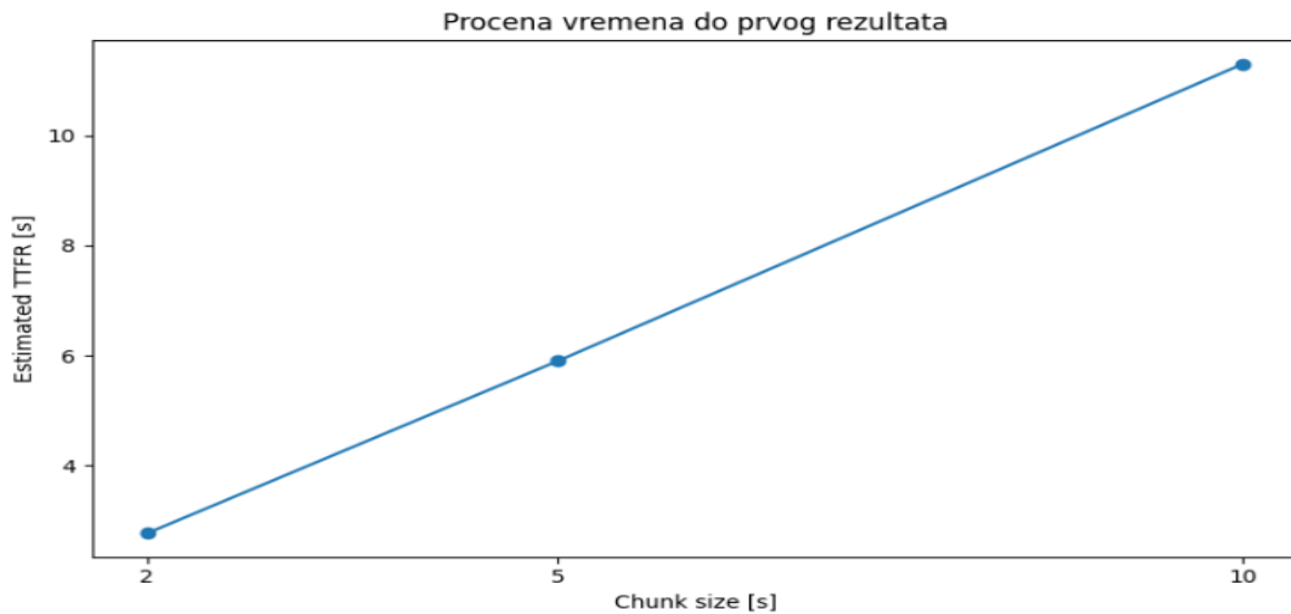
Слика 7. Процена времена до првог резултата
