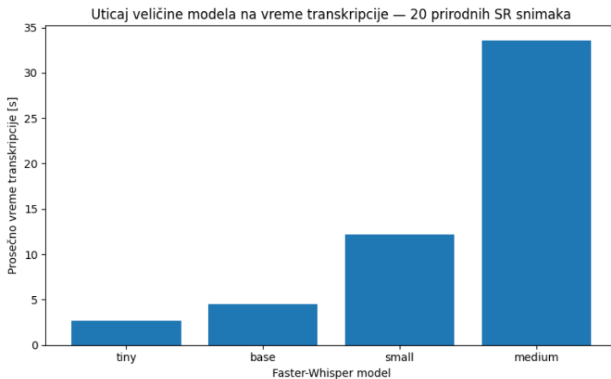
Слика 1. Утицај велићине модела на време транскрипције
