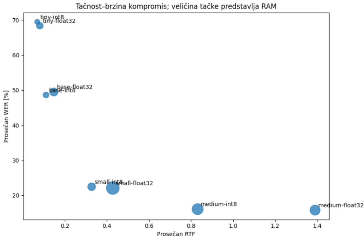
Слика 8. Тачност-брзина компромис
