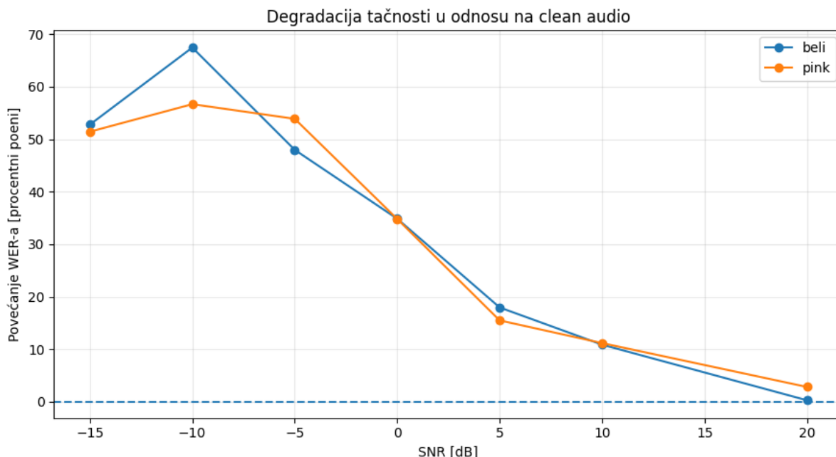
Слика 3. Деградација тачности у доносу на clean audio
