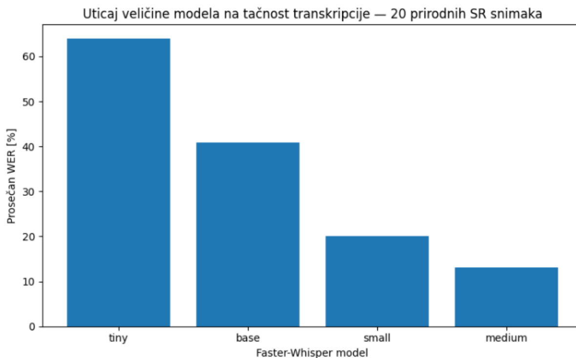
Слика 2. Утицај велићине модела на тачност транскрипције
