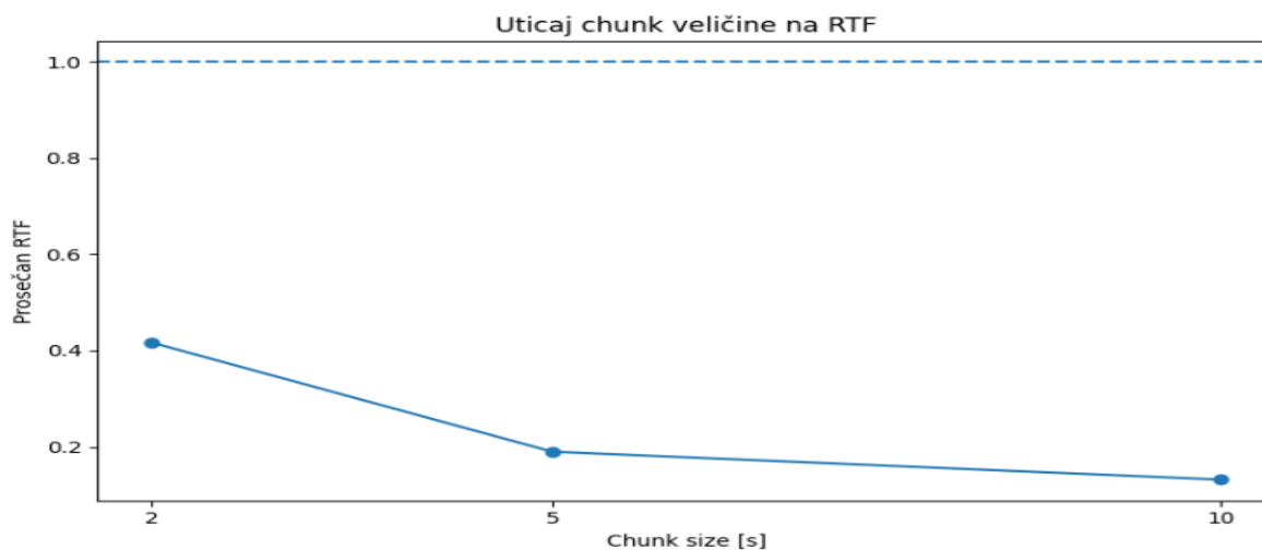
Слика 6. Утицај chunk величине на RTF
